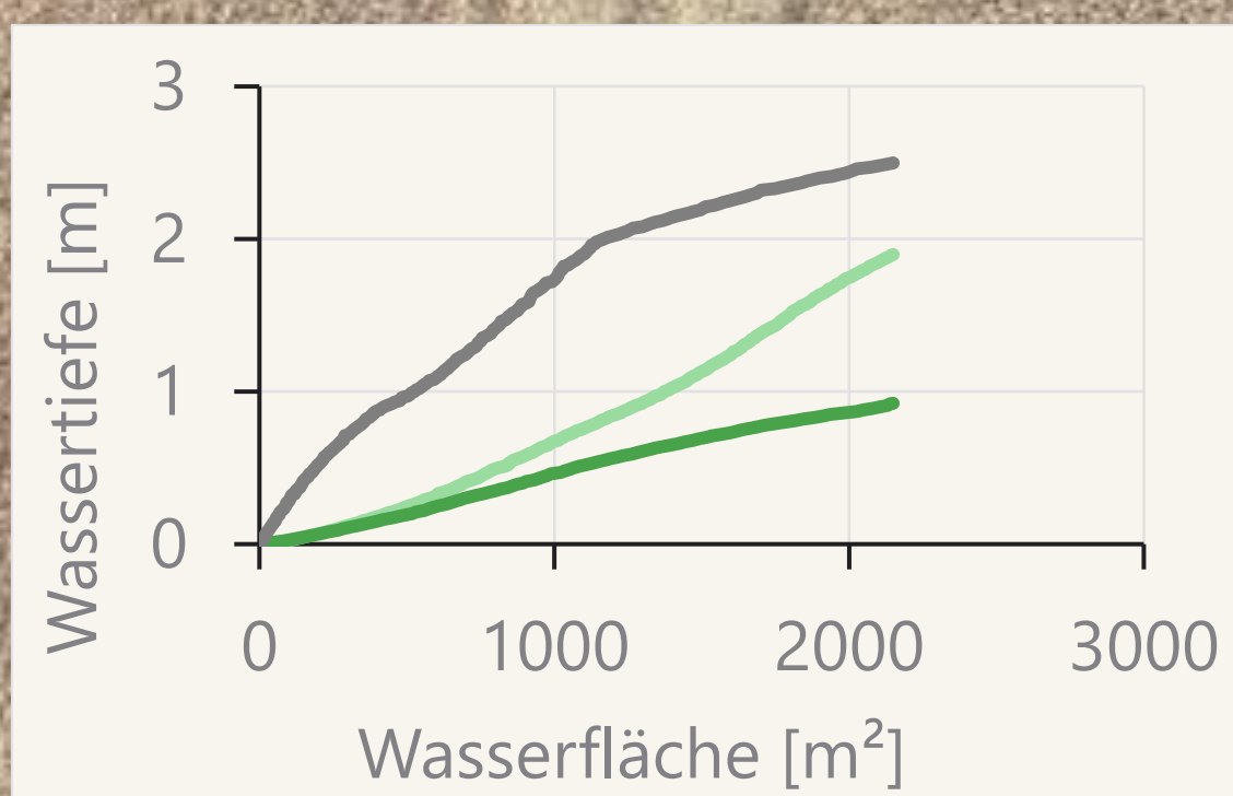
Abb. 1: Aus Regionalisierung bathymetrischer Punktdaten abgeleitetes Verhältnis zwischen Wasserfläche und Wassertiefe drei verschiedener Sölle im Untersuchungsgebiet
