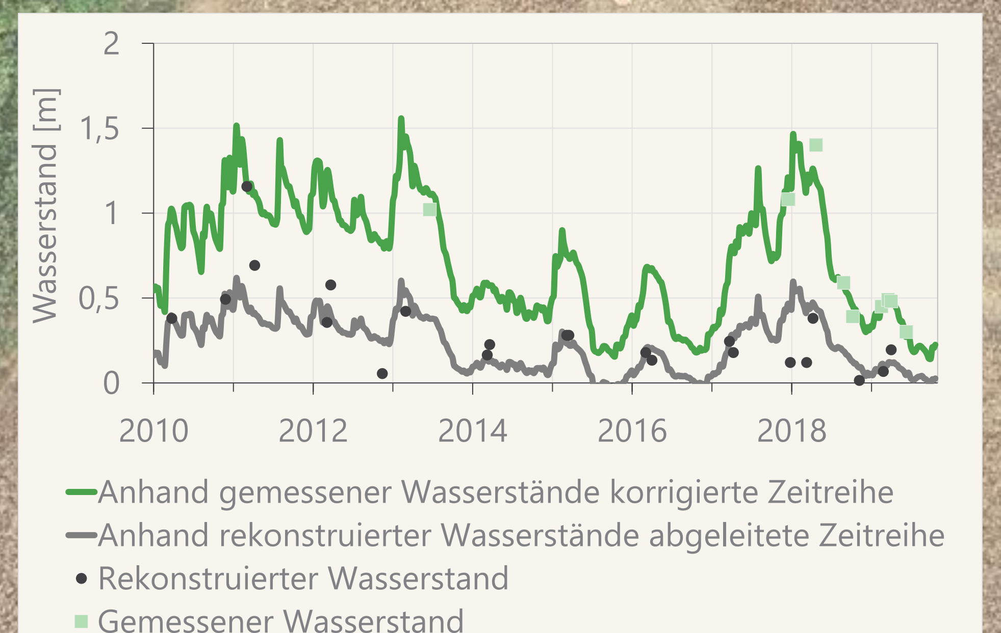
Abb. 2: Rekonstruierte Zeitreihe des Wasserstands für ein Soll auf Basis der vorgestellten Methodik und auf Basis von gemessenen Wasserständen
